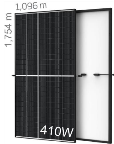
Vertex S (2021) TSM-DE09.08
