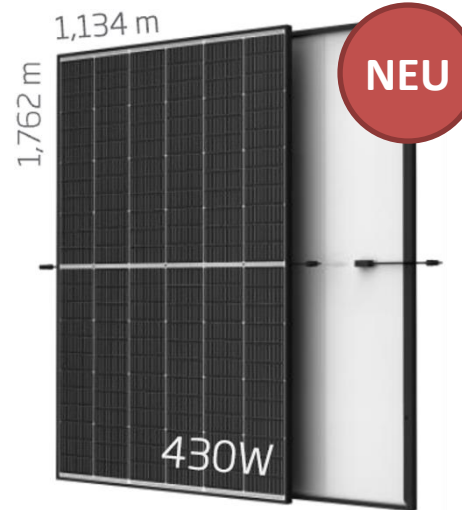
Vertex S (2023) TSM-DE09R.08
